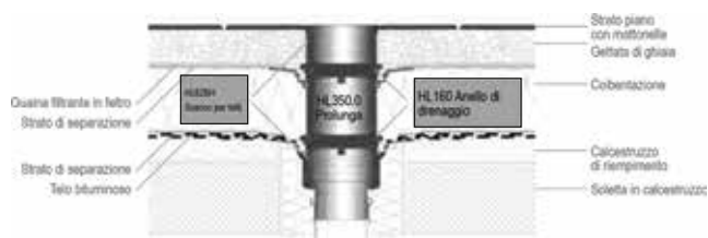
TETTO A TERRAZZA, TETTO COIBENTATO, TETTO ROVESCiato
