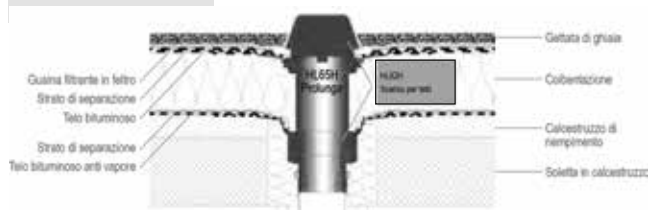
TETTO COIBENTATO CON GETTATA DI GHIAIA
